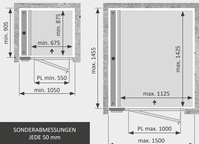
DIMENSIONIERUNG IM MAUERSCHACHT MIN. MAX.
