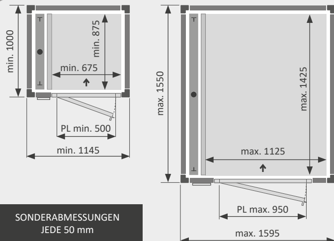
DIMENSIONIERUNG MIT CROSS 50.2 STRUKTUR MIN. MAX.
